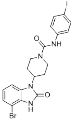
PC-3580601, DMSO-d6
